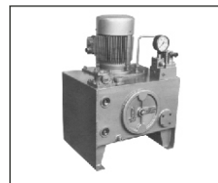
Pogonski agregati 1HAV KONSTRUKCIJA SA ZAVARENIM REZERVOAROM I ZUPČASTOM PUMPOM Hydraulic power units 1 HAV DESIGN WITH WELDED RESERVOIR AND GEAR PUMP
